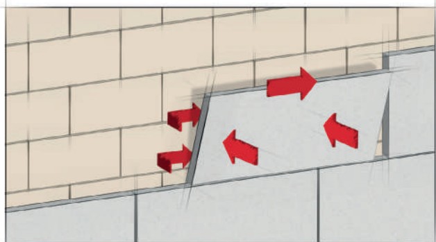
Przyklejanie płyt izolacyjnych
