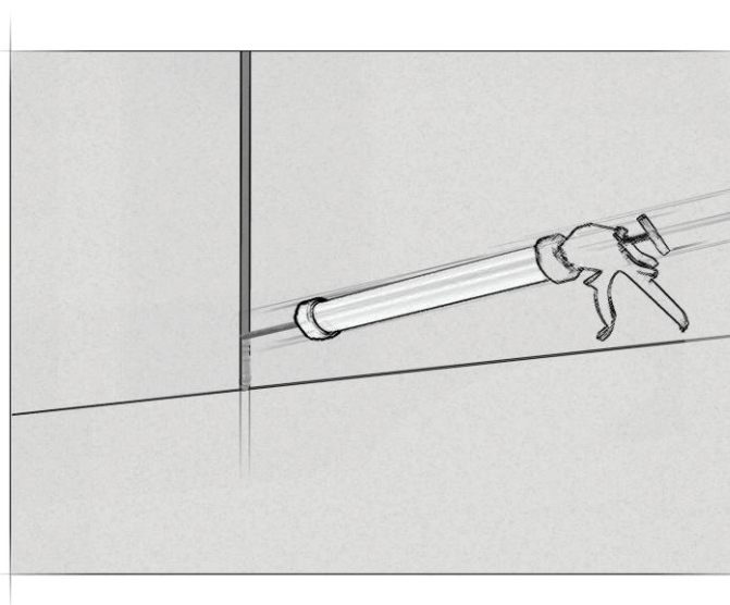
Uzupełnianie pianką poliuretanową szczelin pomiędzy płytami izolacyjnymi
