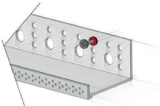
Montaż listwy za pomocą kołków rozporowych
